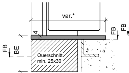
Typ: KSA.B (Alu-Konter-Umbauschwelle)
