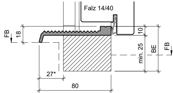
Typ: GS-TT (für Aussentüren) Achtung: Nicht bei Brandschutz- funktion!
