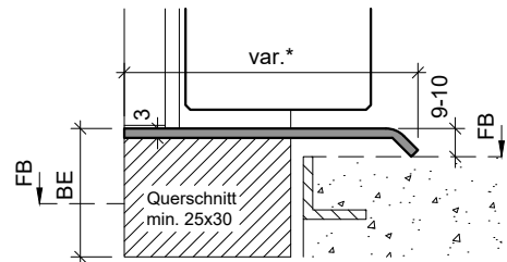
Typ: KSR.B (Alu-Konter-Umbauschwelle)
