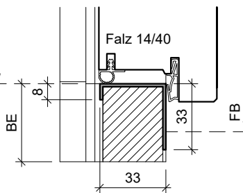
Typ: SP33.B (Abdeckprofil) Edelstahl
