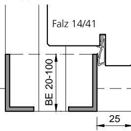
Typ: S+S (Doppelschwelle)
