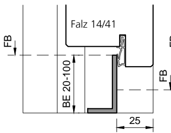
Typ: S (Schwellenwinkel)
