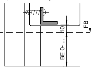
Typ VP (prov. Verbindungsisen)
