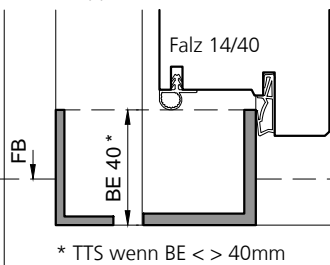
Typ: TT40S+S (Doppelschwelle)
