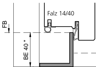
Typ: TT40S (Schwellenwinkel)
