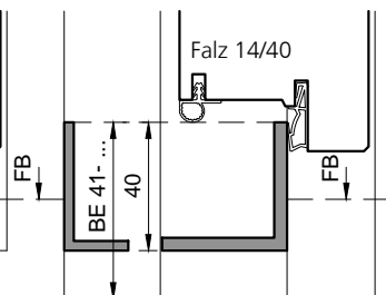
Typ: TT40S+S (Doppelschwelle)
