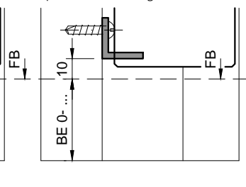
Typ VP (prov. Verbindungseisen)
