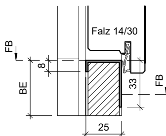
Typ: SP25.B (Abdeckprofil) Edelstahl
