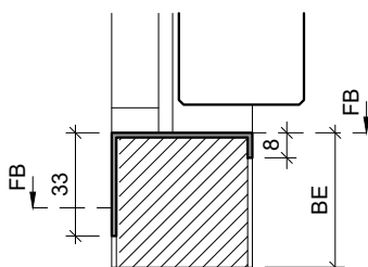
Typ: KSP.B (Sonderanfertigung) (Konter-Abdeckprofil) Edelstahl Breite = Rahmendicke
