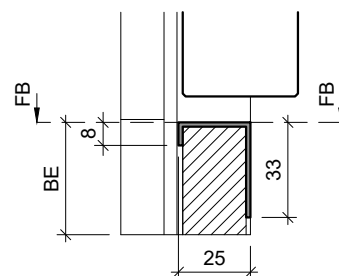
Typ: V-SP25.B (Abdeckprofil) Edelstahl
