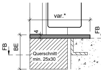
Typ: KSA.B (Alu-Konter-Umbauschwelle)
