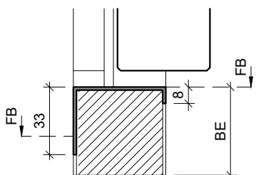
Typ: KSP.B (Sonderanfertigung) (Konter-Abdeckprofil) Edelstahl Breite = Rahmendicke
