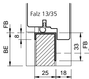
Typ: SP25 (Abdeckprofil) CrNi-Stahl/verzinkt/einbrennlackiert
