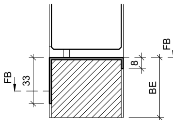
Typ: KSP.B (Sonderanfertigung) (Konter-Abdeckprofil) Edelstahl Breite = Rahmendicke
