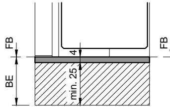
Typ: KSA.B (Alu-Konter-Schwelle) Breite = Rahmendicke
