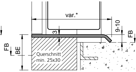
Typ: KSR.B (Alu-Konter-Umbauschwelle)
