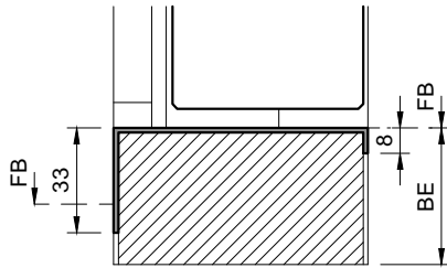
Typ: KSP.B (Sonderanfertigung) (Konter-Abdeckprofil) CrNi-Stahl/verzinkt/einbrennlackiert Breite = Rahmendicke
