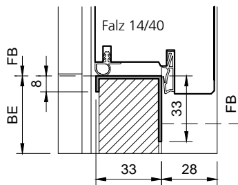
Typ: SP33 (Abdeckprofil) CrNi-Stahl/verzinkt/einbrennlackiert
