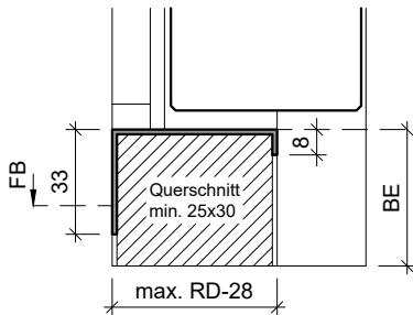
Typ: KSP.B (Sonderanfertigung) (Konter-Abdeckprofil) Edelstahl
