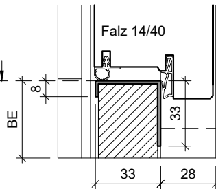
Typ: SP33 (Abdeckprofil) Edelstahl
