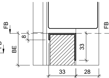
Typ: V-SP33 (Abdeckprofil) Edelstahl
