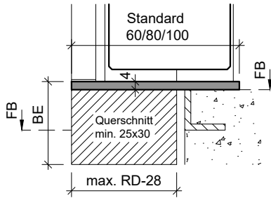
Typ: KSP.B (Sonderanfertigung) (Konter-Abdeckprofil) Edelstahl
