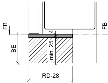
Typ: KSA.B (Alu-Konter-Schwelle) Schwellenbreite = Holzdicke
