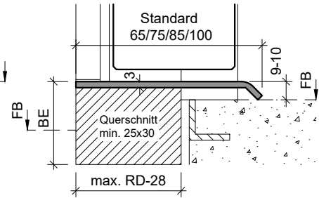
Typ: V-SP33 (Abdeckprofil) Edelstahl
