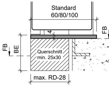
Typ: KSP.B (Sonderanfertigung) (Konter-Abdeckprofil) Edelstahl
