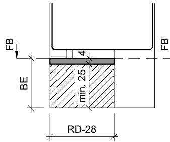
Typ: KSA.B (Alu-Konter-Schwelle) Schwellenbreite = Holzdicke
