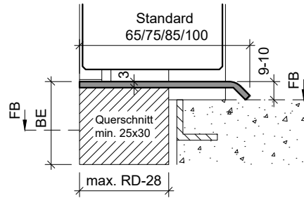
Typ: V-SP33 (Abdeckprofil) Edelstahl
