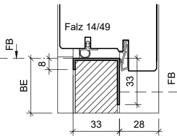
Typ: SP33 (Abdeckprofil) Edelstahl
