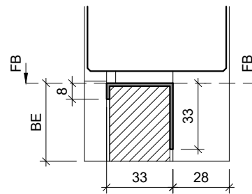
Typ: V-SP33 (Abdeckprofil) Edelstahl
