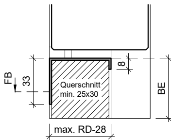
Typ: KSP.B (Sonderanfertigung) (Konter-Abdeckprofil) Edelstahl
