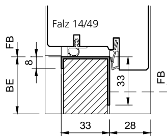
Typ: SP33 (Abdeckprofil) CrNi-Stahl/verzinkt/einbrennlackiert
