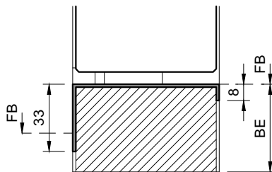
Typ: KSP.B (Sonderanfertigung) (Konter-Abdeckprofil) CrNi-Stahl/verzinkt/einbrennlackiert Breite = Rahmendicke
