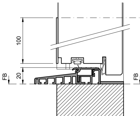
Schnitt Türblatt
