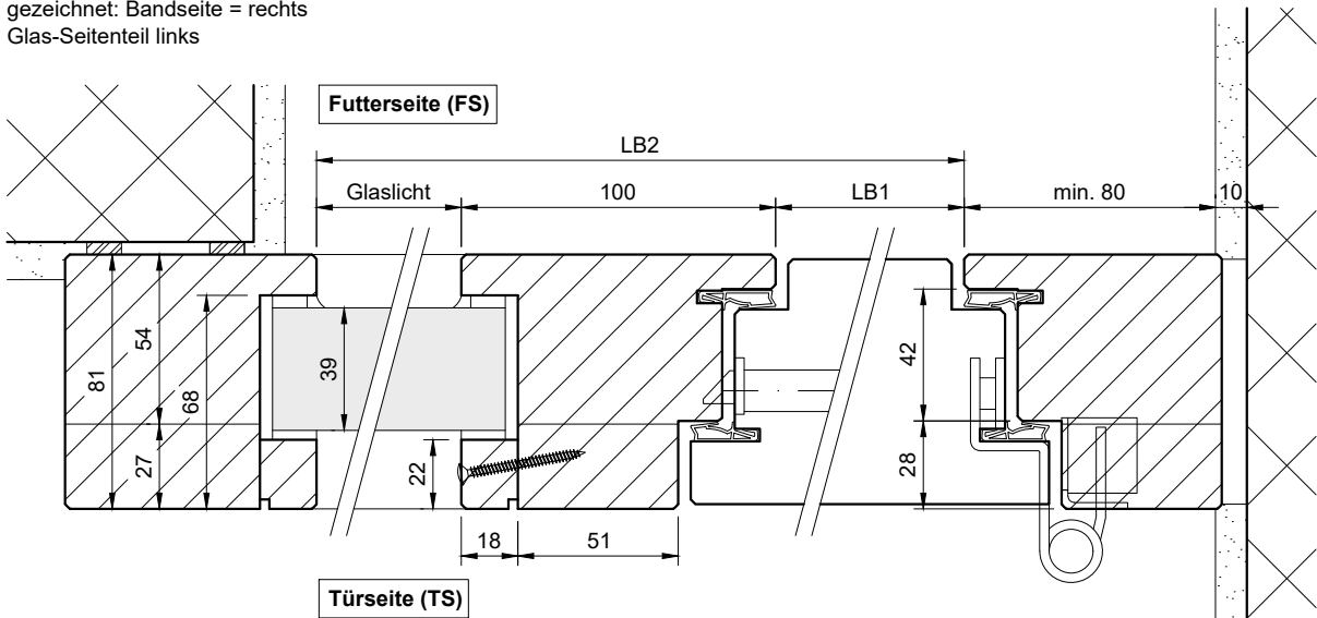
Schnitt Türblatt
