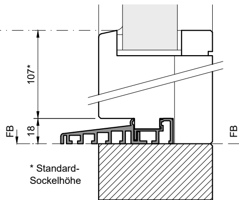
Schnitt Glas-Seitenteil
