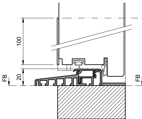
Schnitt Türblatt
