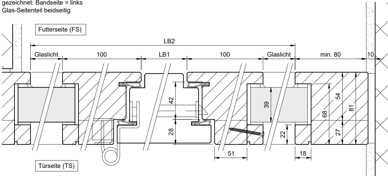
Schnitt Türblatt
