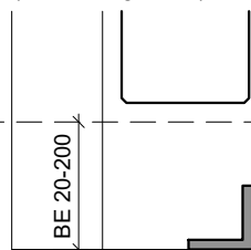
Typ: V (Verbindungseisen)
