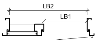
Band rechts, Glas-Seitenteil links (Keller Z. Variante C)
