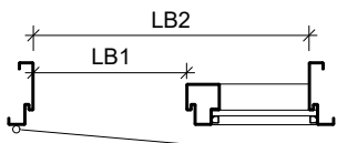
Band links, Glas-Seitenteil rechts (Keller Z. Variante A)
