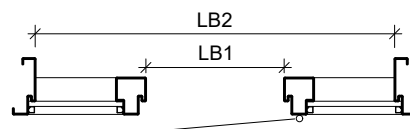
Band rechts, Glas-Seitenteil beidseitig
