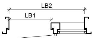
Band rechts, Glas-Seitenteil rechts (Keller Z. Variante B)
