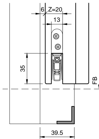
Typ: TTD39 49-61mm Türblatt
