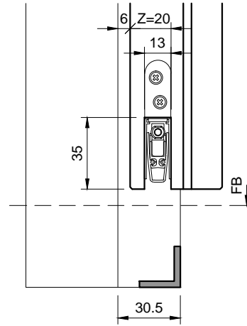
Typ: TTD30 43-52mm Türblatt
