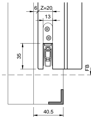
Typ: TTD40 58-61mm Türblatt
