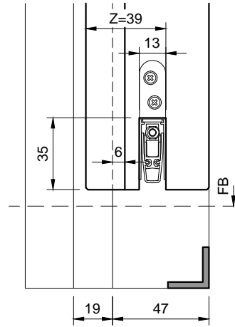
Typ: UDDS 58-61mm Türblatt (Zusatzfalz = 19mm)
