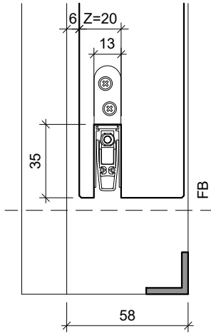
Typ: UDS58 49-50mm Türblatt
