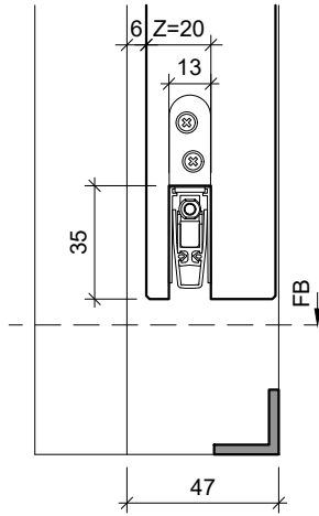
Typ: TTUDS 39-41mm Türblatt
