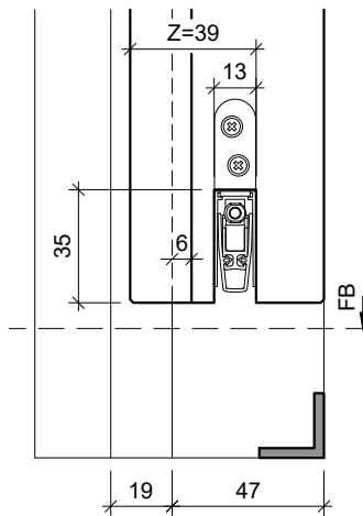
Typ: UDDS 58-61mm Türblatt (Zusatzfalz = 19mm)
