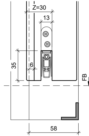
Typ: UDS58 58-61mm Türblatt (Zusatzfalz = 9mm)
