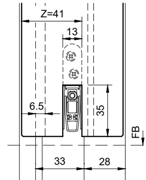
Stehflügel (Schnitt)
