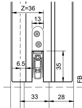
Gehflügel (Ansicht)
