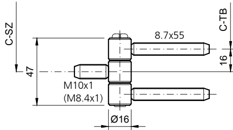
16-3.Z (SZ) blau/weiss verzinkt
