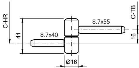
16-2B.R (HR) blau/weiss verzinkt
