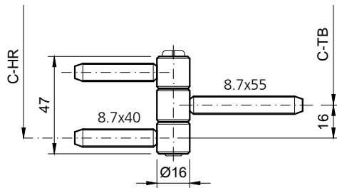
16-3B.R (HR) blau/weiss verzinkt
