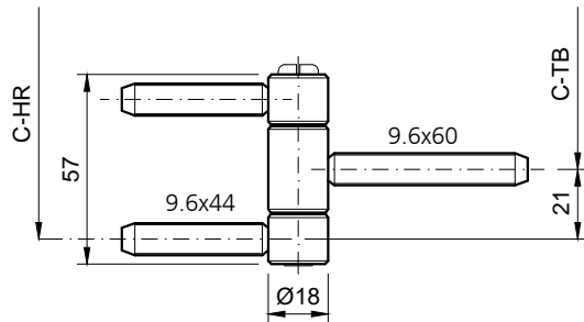
18-3B.R (HR) blau/weiss verzinkt
