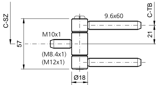
HE18 (SZ) blau/weiss verzinkt
