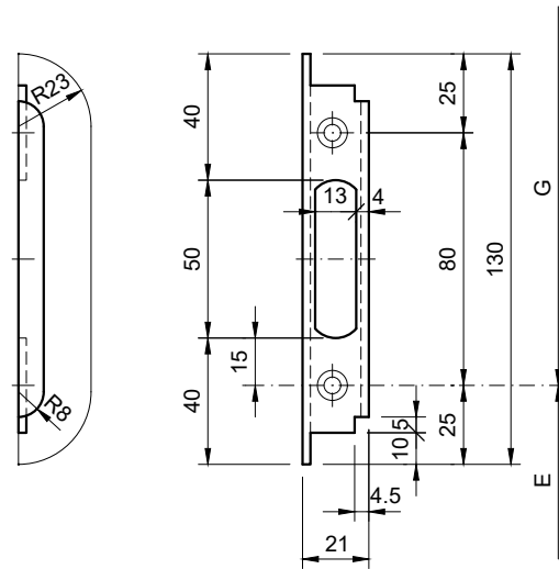
Typ: Koch 67.337.62 (Edelstahl) Einfräs-Fallenschliessblech für Glastüren
