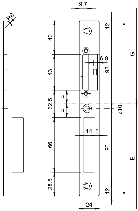
Typ: V-1133.6-9 (Edelstahl) Kappenschliessblech
