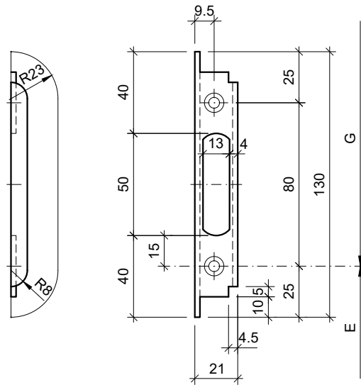
Typ: Koch 67.161.532 (Edelstahl) Einfräs-Fallenschliessblech für Glastüren
