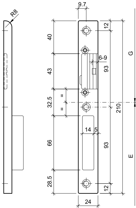
Typ: V-1133.6-9 (Edelstahl) Kappenschliessblech
