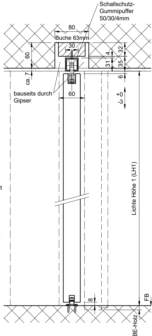
HAWA Adapto 80 Beschlag: Junior 80/B-Pocket
