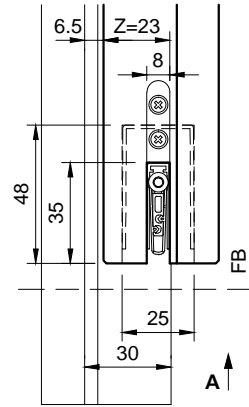
Typ: RD17-30 38-50mm Türblatt
