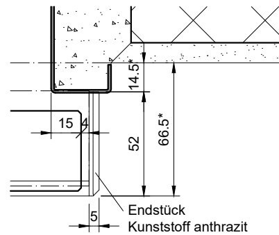
Schlosseite, Detail (S1)
