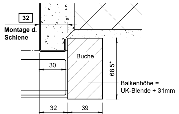
mit Einlaufbalken, Detail (S2)
