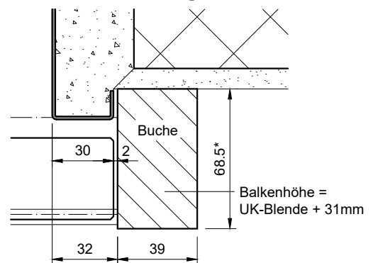
mit Einlaufbalken, Detail (S2)
