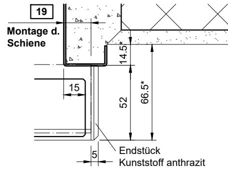
Schlosseite, Detail (S1)
