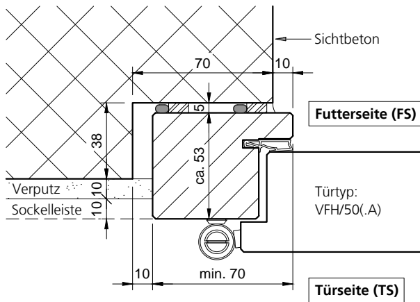
Typ RD17-40, Variante 2 Futterseite Sichtbeton, Türseite verputzt
