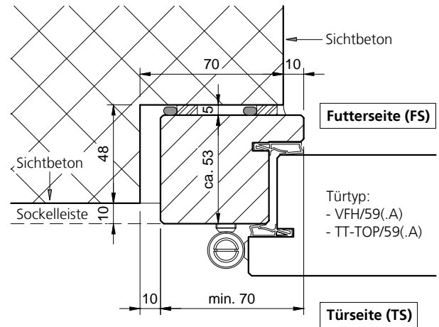
Typ RD17-40, Variante 1 Futter- und Türseite Sichtbeton
