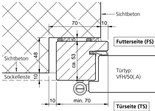
Typ RD17-40, Variante 1 Futter- und Türseite Sichtbeton
