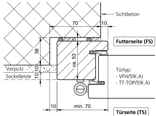
Typ RD17-40, Variante 2 Futterseite Sichtbeton, Türseite verputzt
