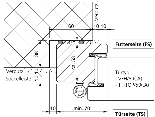
Typ RD17-40, Variante 3 Futter- und Türseite verputzt
