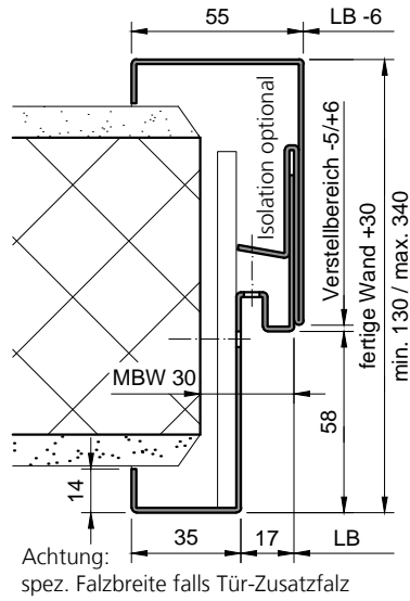
Steckzarge (ST-...-GL)
