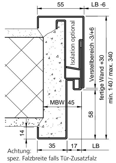
Steckzarge (ST-...-GL-ZP)
