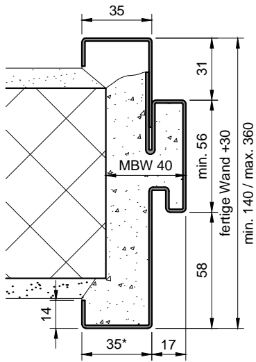
Steckzarge (ST-...-BF)
