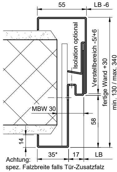
Steckzarge (ST-...-GL)
