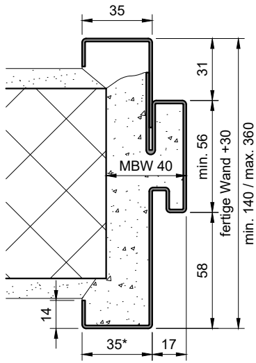
Steckzarge (ST-...-BF)
