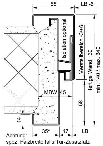
Steckzarge (ST-...-GL-ZP)
