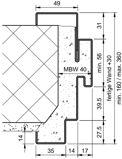
Steckzarge (ST-...-BF)
