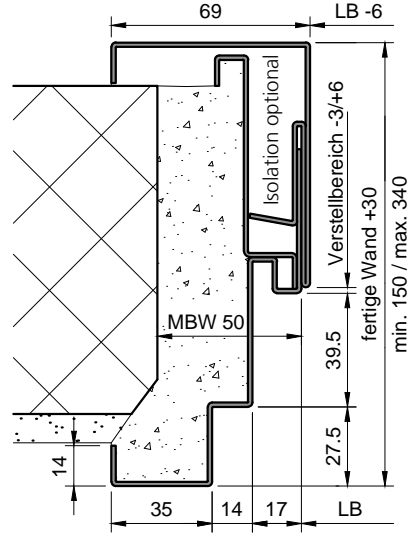
Steckzarge (ST-...-GL-ZP)
