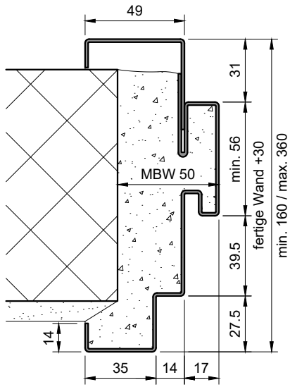
Steckzarge (ST-...-BF)
