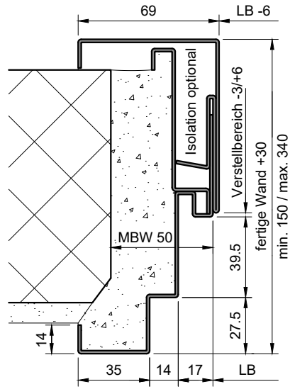
Steckzarge (ST-...-GL-ZP)
