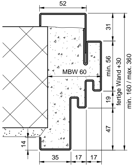
Steckzarge (ST-...-BF)
