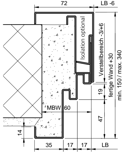
Steckzarge (ST-...-GL-ZP)
