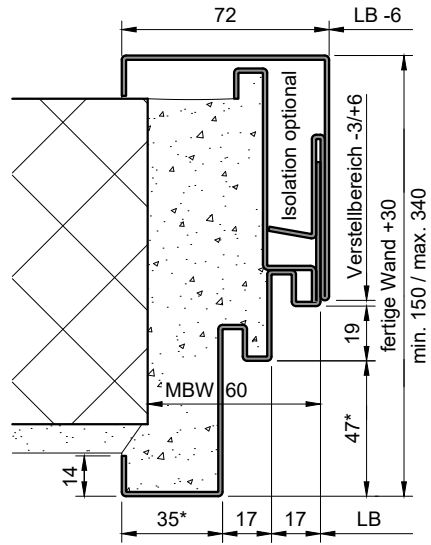
Steckzarge (ST-...-GL-ZP)
