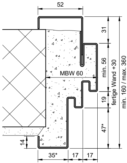
Steckzarge (ST-...-BF)
