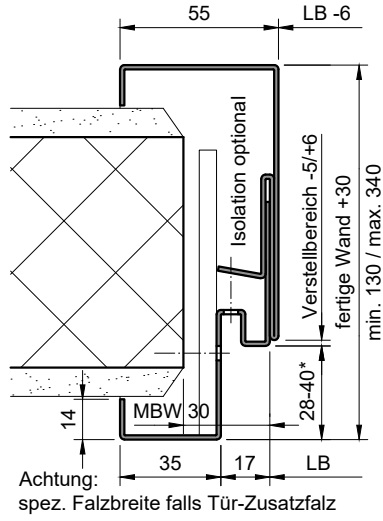
Steckzarge (ST-...-GL)
