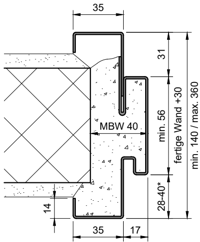
Steckzarge (ST-...-BF)
