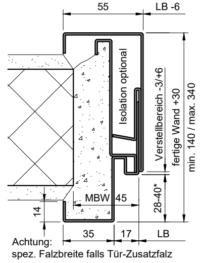
Steckzarge (ST-...-GL-ZP)
