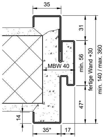
Steckzarge (ST-...-BF)
