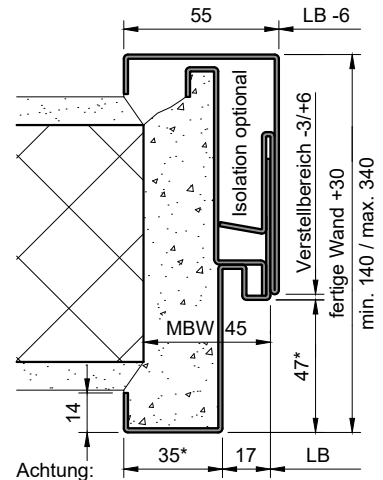
Steckzarge (ST-...-GL-ZP)
