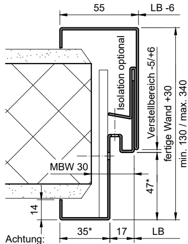
Steckzarge (ST-...-GL)
