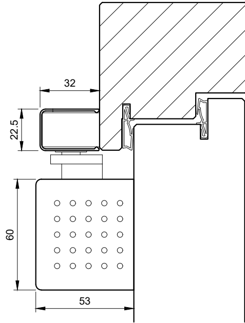
Türblattmontage Futterseite mit Sturzfutterwinkel
