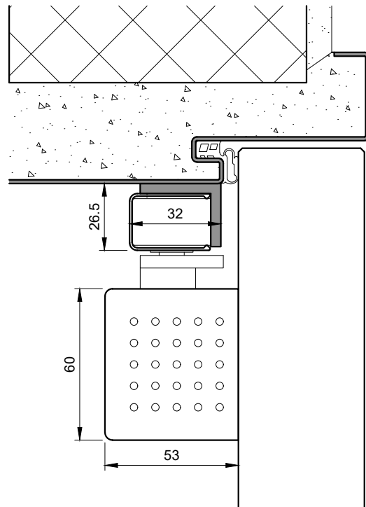
Türblattmontage Futterseite mit Sturzfutterwinkel
