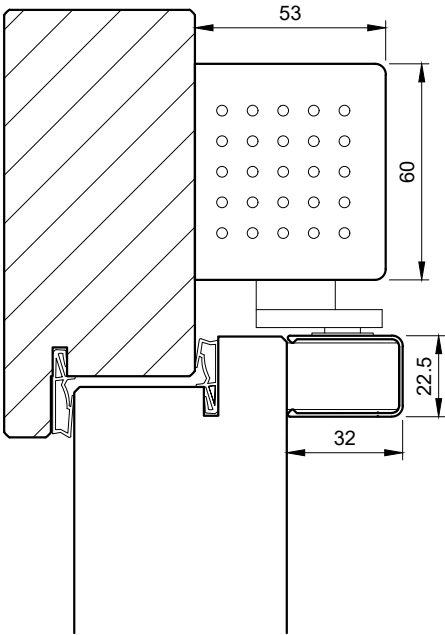
Kopf- /Sturzmontage Türseite
