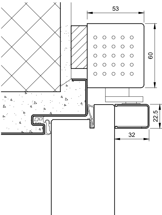
Kopf- /Sturzmontage Türseite
