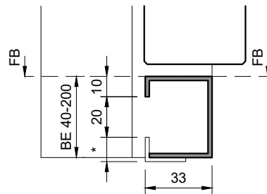
Stahlzarge TTD39, Bodenverbindung VSP33 KZA: CNS-SP33
