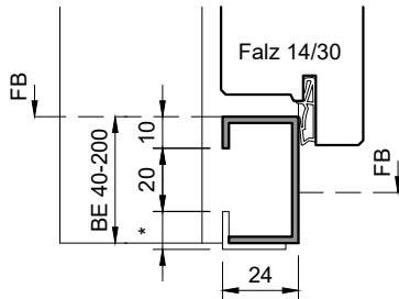
Stahlzarge TTD30, Schwellenprofil ZSP24 KZA: CNS-SP24
