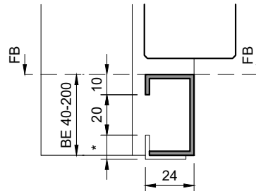
Stahlzarge TTD30, Bodenverbindung VSP24 KZA: CNS-SP24
