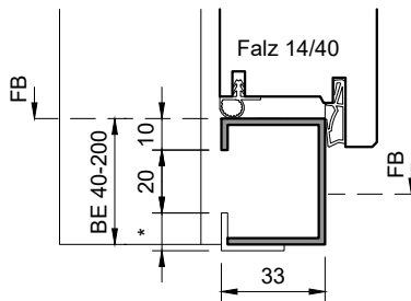
Stahlzarge TTD39, Schwellenprofil ZSP33 KZA: CNS-SP33
