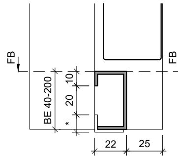
Stahlzarge UDS58, Bodenverbindung VSP26 KZA: CNS-SP26
