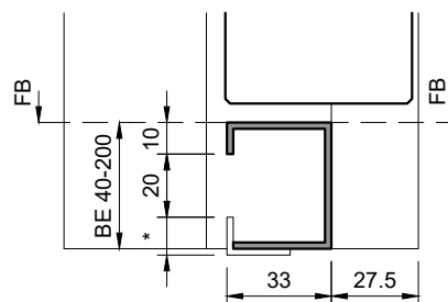
Stahlzarge UDS27/39, Bodenverbindung VSP33 KZA: CNS-SP33
