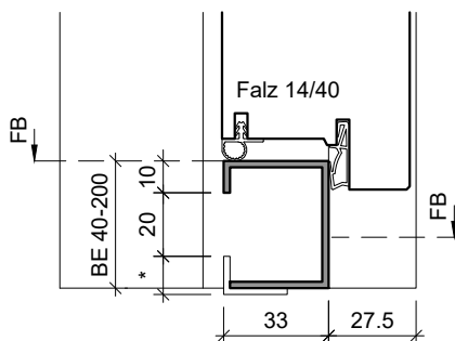
Stahlzarge UDS27/39, Schwellenprofil ZSP33 KZA: CNS-SP33
