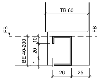
Stahlzarge UDS58, Bodenverbindung VSP26 KZA: CNS-SP26
