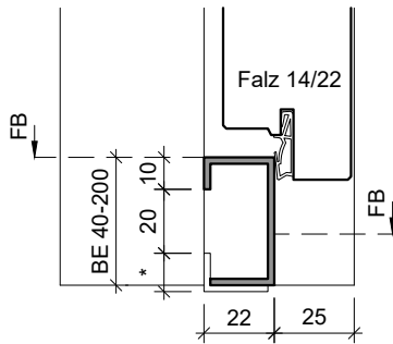
Stahlzarge UDS58, Schwellenprofil ZSP26 KZA: CNS-SP26
