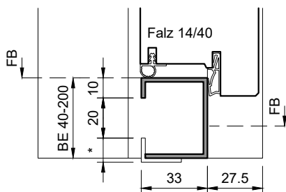
Stahlzarge UDS27/39, Schwellenprofil ZSP33 KZA: CNS-SP33
