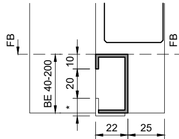
Stahlzarge TTUDS, Bodenverbindung VSP22 KZA: CNS-SP22
