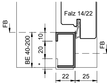
Stahlzarge TTUDS, Schwellenprofil ZSP22 KZA: CNS-SP22
