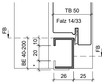
Stahlzarge UDS58, Schwellenprofil ZSP26 KZA: CNS-SP26
