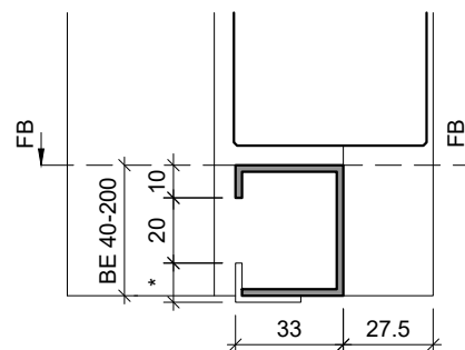
Stahlzarge UDS27/39, Bodenverbindung VSP33 KZA: CNS-SP33
