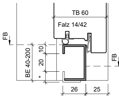
Stahlzarge UDS58, Schwellenprofil ZSP26 KZA: CNS-SP26
