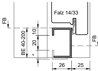
Stahlzarge UDS58, Schwellenprofil ZSP26 KZA: CNS-SP26
