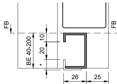
Stahlzarge UDS58, Bodenverbindung VSP26 KZA: CNS-SP26
