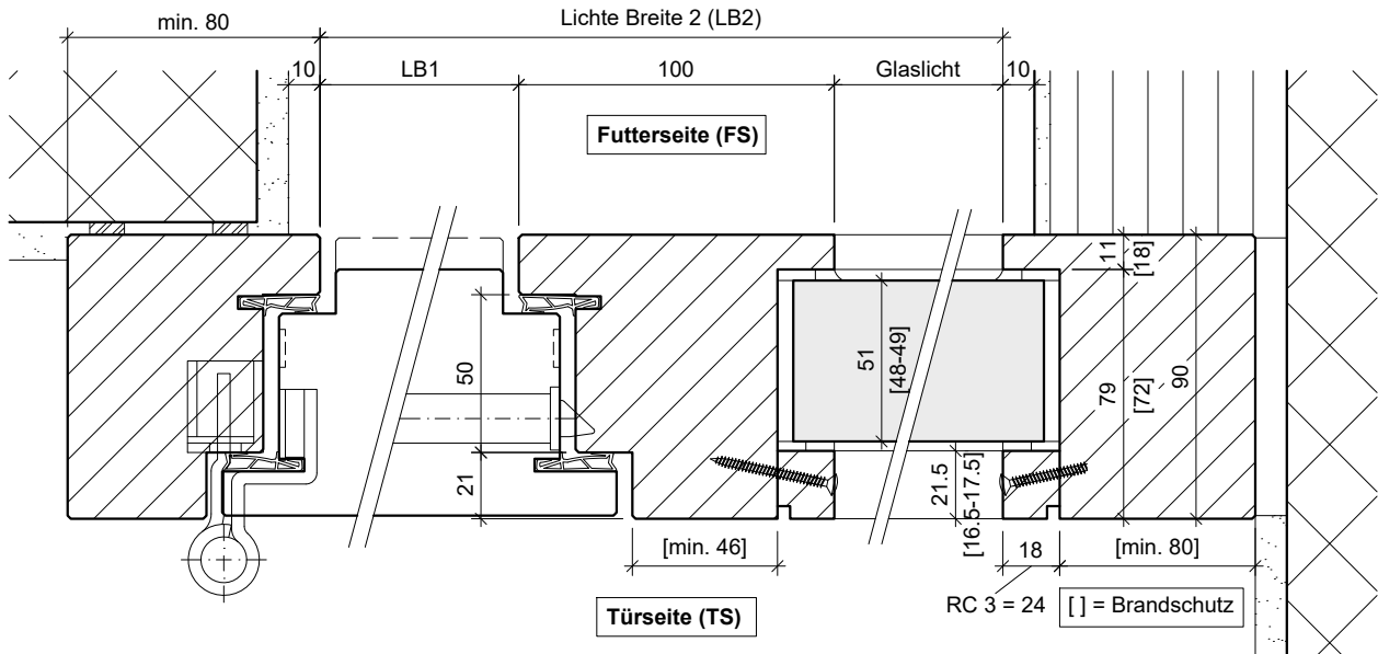
Schnitt TB mit Sockelblech
