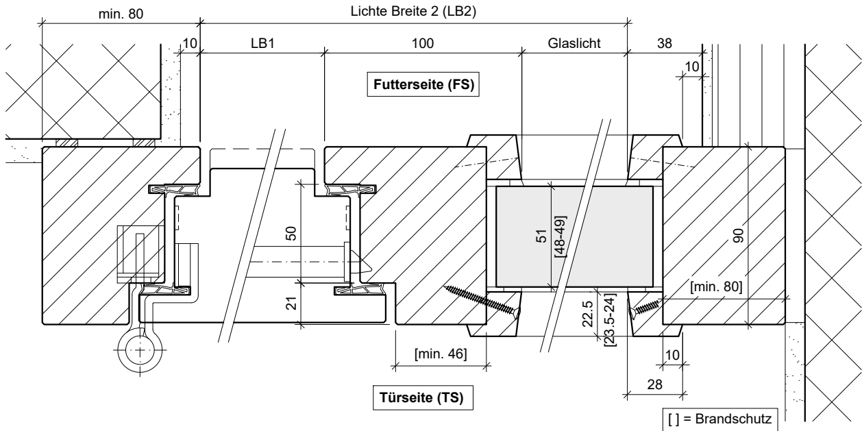
Schnitt TB mit Sockelblech
