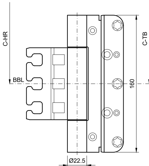
VX 7859/FD/160 15/5 (HR) Edelstahl matt
