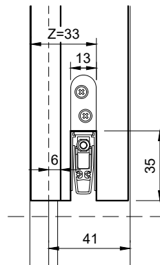
Gehflügel (Ansicht)
