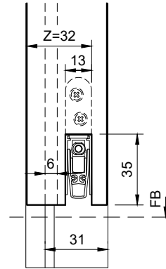
Stehflügel (Schnitt)
