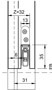
Gehflügel (Ansicht)
