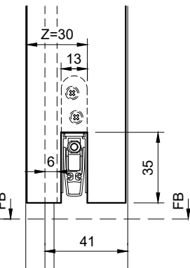
Stehflügel (Schnitt)
