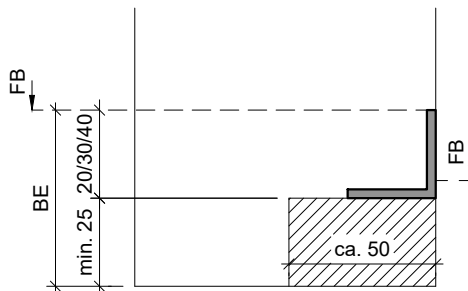
Typ: KSW.B (Konterschwellen)
