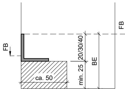
Typ: KSW.B (Konterschwellen)
