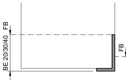
Typ: SW.B (Schwellenwinkel)
