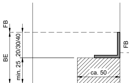
Typ: KSW.B (Konterschwelle)
