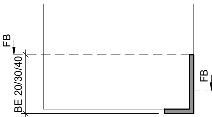
Typ: SW.B (Schwellenwinkel)
