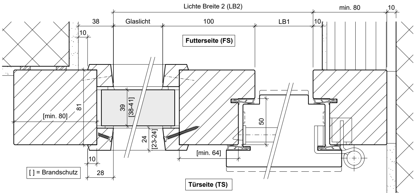
Schnitt TB mit Sockelblech
