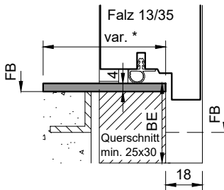
Typ: SA (Alu-Umbauschwelle)
