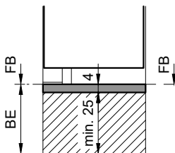
Typ: KSA.B (Alu-Konter-Schwelle) Breite = Rahmendicke
