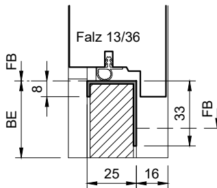
Typ: SP25 (Abdeckprofil) Edelstahl
