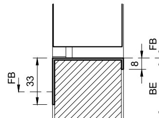
Typ: KSP.B (Sonderanfertigung) (Konter-Abdeckprofil) Edelstahl Breite = Rahmendicke
