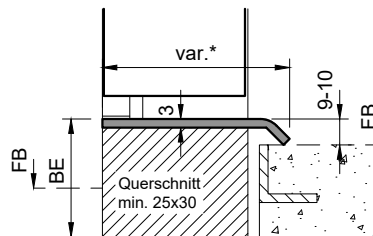
Typ: KSR.B (Alu-Konter-Umbauschwelle)
