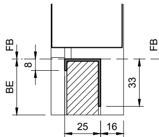
Typ: V-SP25 (Abdeckprofil) Edelstahl
