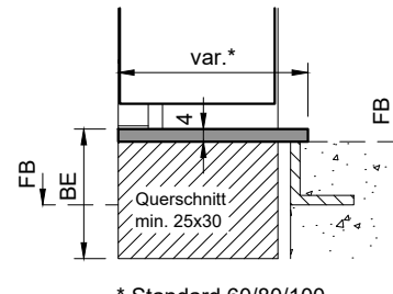
Typ: KSA.B (Alu-Konter-Umbauschwelle)
